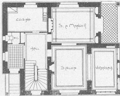
Plan du rez-de-chaussée. Echelle 1 : 200.
