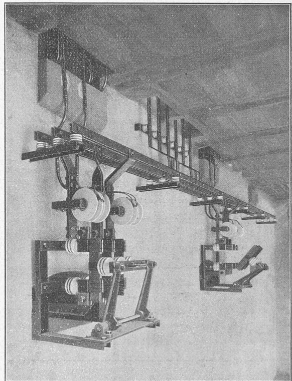
Fig. 18. — Barres collectrices secondaires avec transformateurs de courant et pièces de connexion amovibles.
