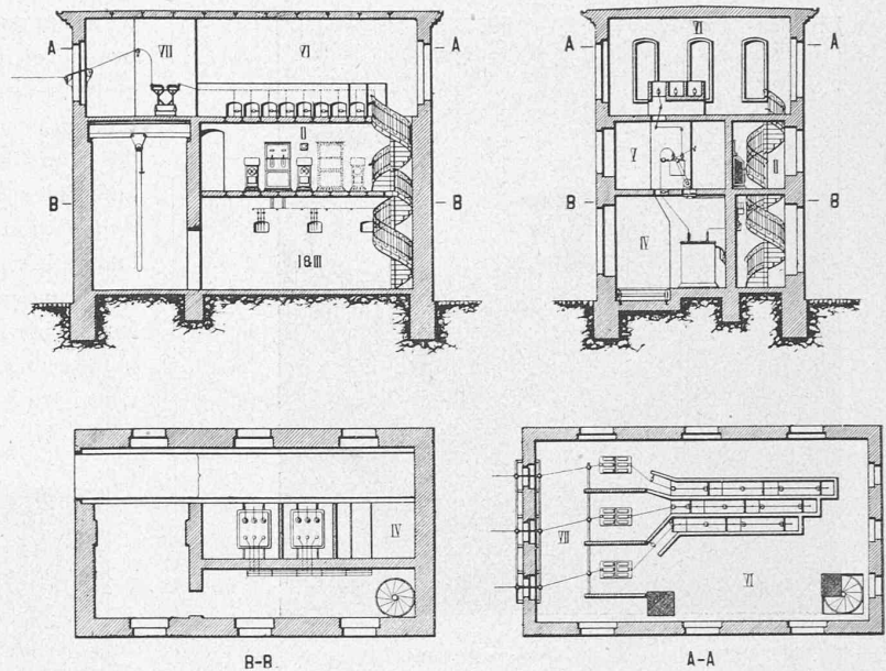
Fig. 49. — Plan et coupes de la station réceptrice de Nembro.
