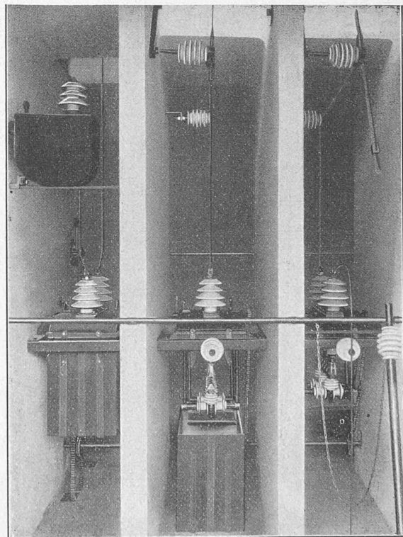
Fig. 9. — Vue de face des interrupteurs automatiques.
