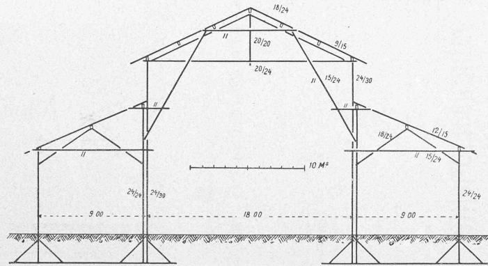
Fig. 4. — Halle des concerts de la fête fédérale de chant de Zurich, en 1880. Distance des fermes : 6 m.
