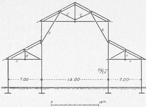
Fig. 1. — Halle de l'exposition cantonale de Zurich, en 1894 1 .
