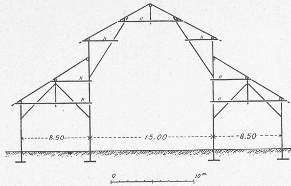
Fig. 3. — Cantine du tir fédéral de Stanz, en 1861.
