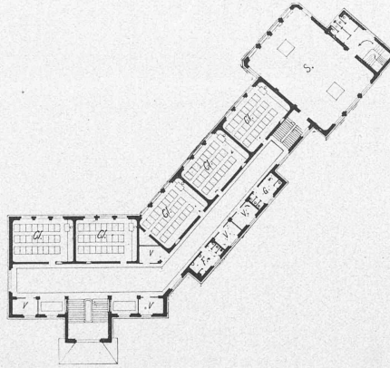
Plan du 1 er étage.
