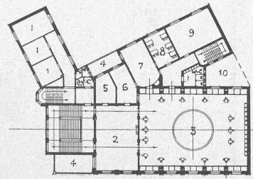
Plan du I er étage.
