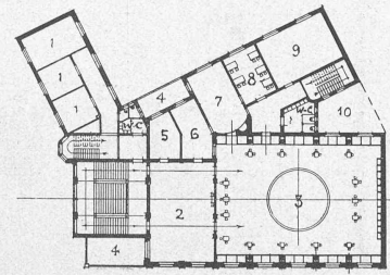
Plan du I er étage.
