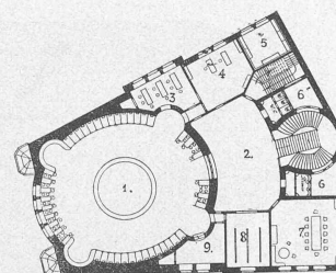
Plan du I er étage.
