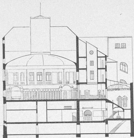
Coupe en long.
