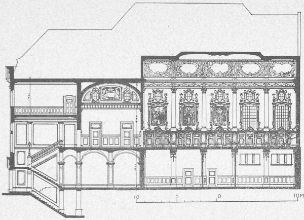
Coupe en long sur AB.
