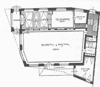
Plan du rez-de-chaussée. — 1 : 500.
