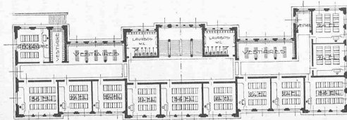
Plan du 2 nd étage. — 1 : 800.
