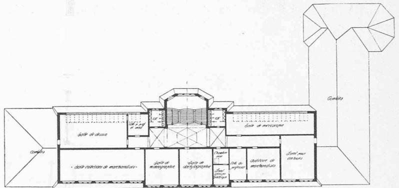
Plan des combles. — 1 : 800.
