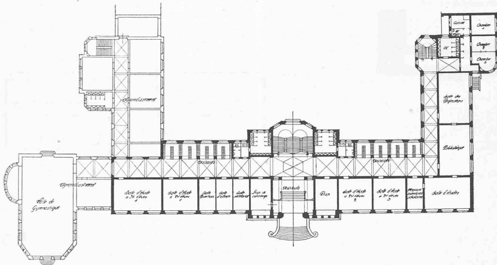
Plan du rez-de-chaussée. — 1 : 800.
