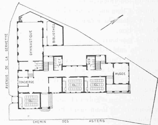
Rez-de-chaussée. — 1 : 1000.
