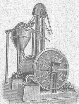
Doppelhartumhle.
