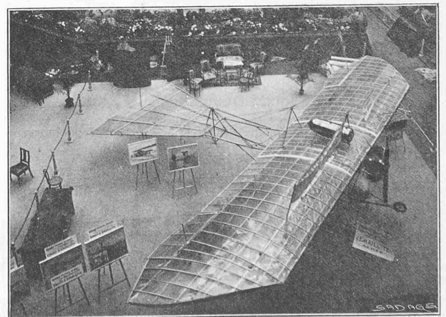
Fig. 2. — L'aérostable Moreau .
