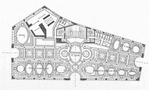
Plan de l'entresol. — 1 : 600.
