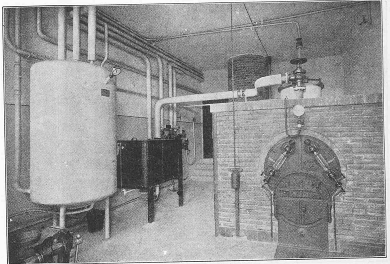
Fig. 6. — Salle des chaudières. (Chaufferie)
