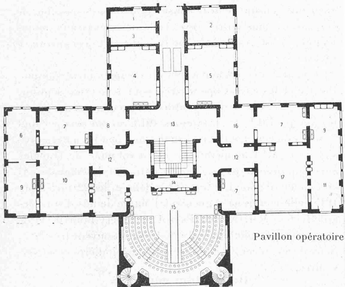
Plans des deuxième étages. — 1 : 500.
