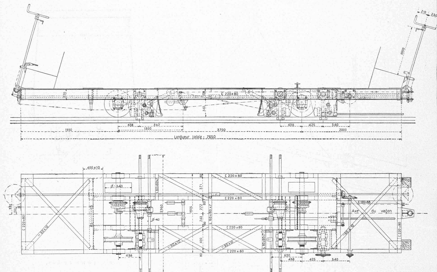
Fig. 26. — Châssis de la voiture-voyageurs. — 1 : 40.
