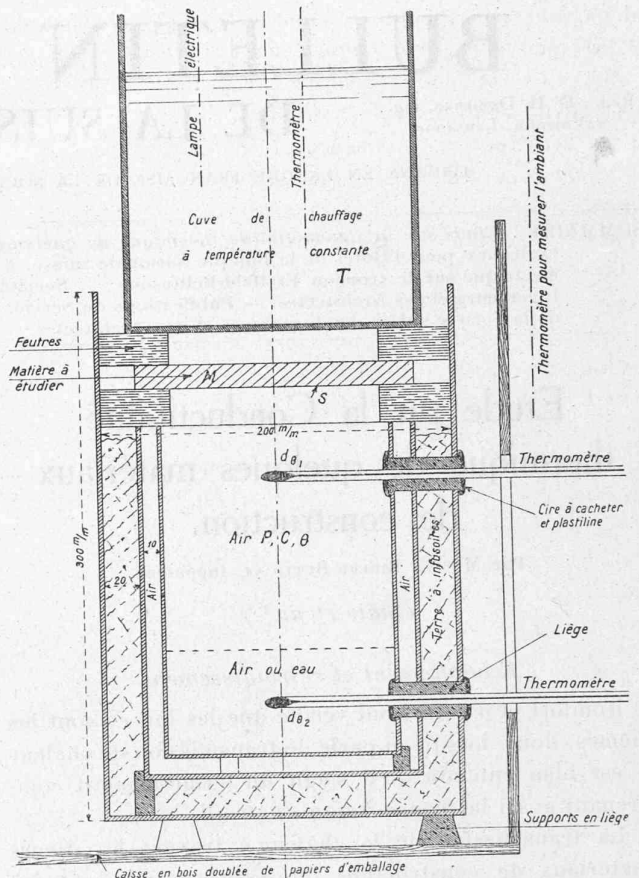
Fig. 4. — Appareil utilisé pour déterminer les coefficients de conductibilité thermique. Température ambiante constante.
