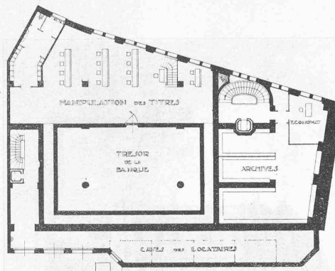
Plan du 1 er sous-sol. — 1 : 800.
