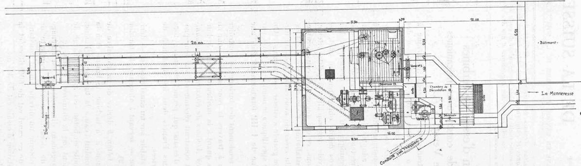
Fig. 1. — Station d'essais des Ateliers de constructions mécaniques de Vevey. Plan général. — 4 : 200.
