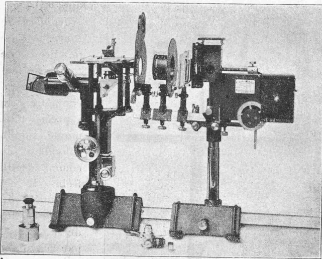
Fig. 32. — Microscope Leitz. Agencement pour les faibles grossissements.
