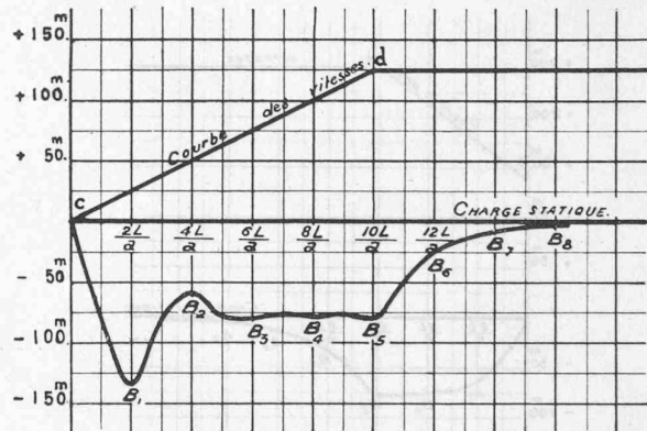
Fig. 17. — Ouverture cd de v_0 = 0 à V_f = 7^m,50 en 10 sec. \frac{aV_f}{2gy_0} > 1 (Basses chutes).
