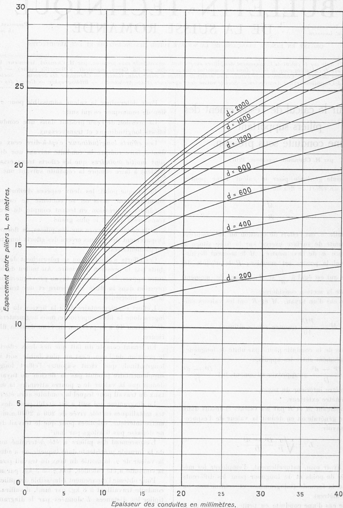
Diagramme donnant l'espacement admissible des piliers supportant une conduite sous pression calculée pour un travail maximum en pleine tôle de 6 kg. par mm 2 .
