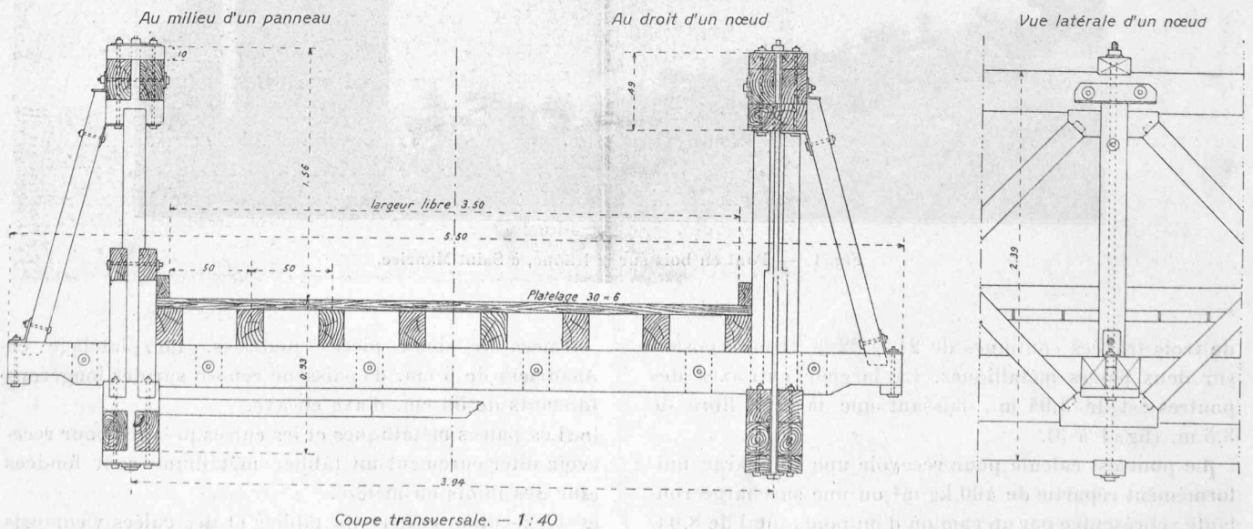
Fig. 3. — Pont en bois sur le Rhône, à Saint-Maurice.
