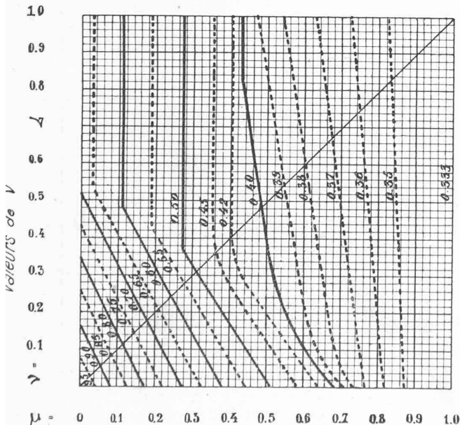
Fig. 14. — Conduites en trois tronçons. Coefficient N du coup de bélier maximum pour fermeture à l'allure \frac{V'}{T} m/sec.
