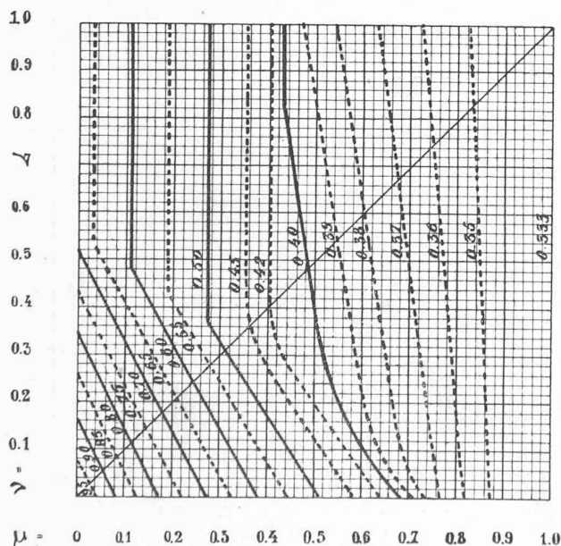
Fig. 14. — Conduites en trois tronçons. Coefficient N du coup de bélier maximum pour fermeture
