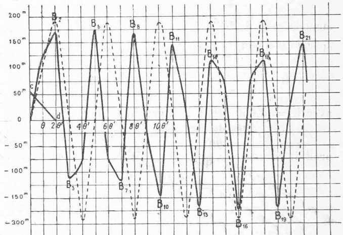
Fig. 4. — Conduites en deux tronçons. Coup de bélier au vannage pour fermeture complète cd
