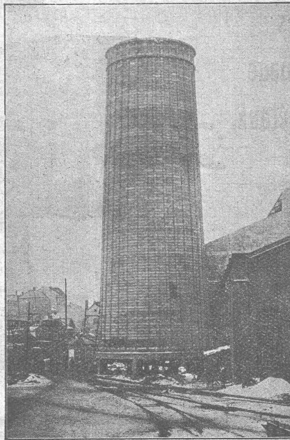
Réfrigérant de 32 m. de hau eur.
