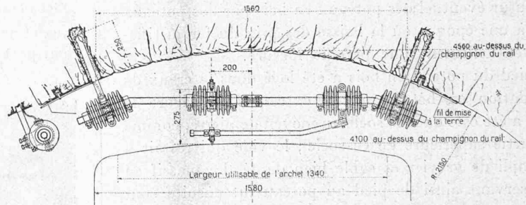
Fig. 6. — Point d'appui en tunnel en rampe. — 1 : 25.
