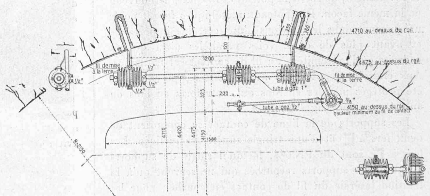
Fig. 7. — Point d'appui de la ligne de contact dans le tunnel de l'Albula. — 1 : 25.
