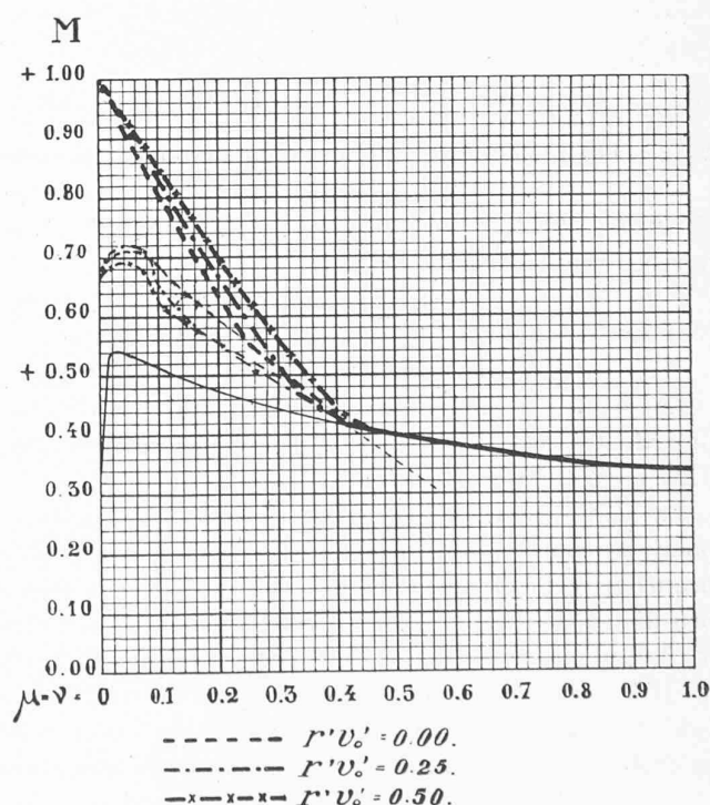
Fig. 11. — Conduites en trois tronçons avec \mu = \gamma . Coefficient M du coup de bélier maximum de fermeture à l'allure
