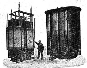
TRANSFORMATEUR MONOPHASE 5000 kVA 60 000/15 000 v. 16 2/3 pér. Fourni aux C.F.F. pour la sous-station de Giubiasco.
