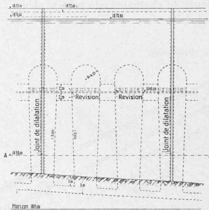
Fig. 9. — Elévation
