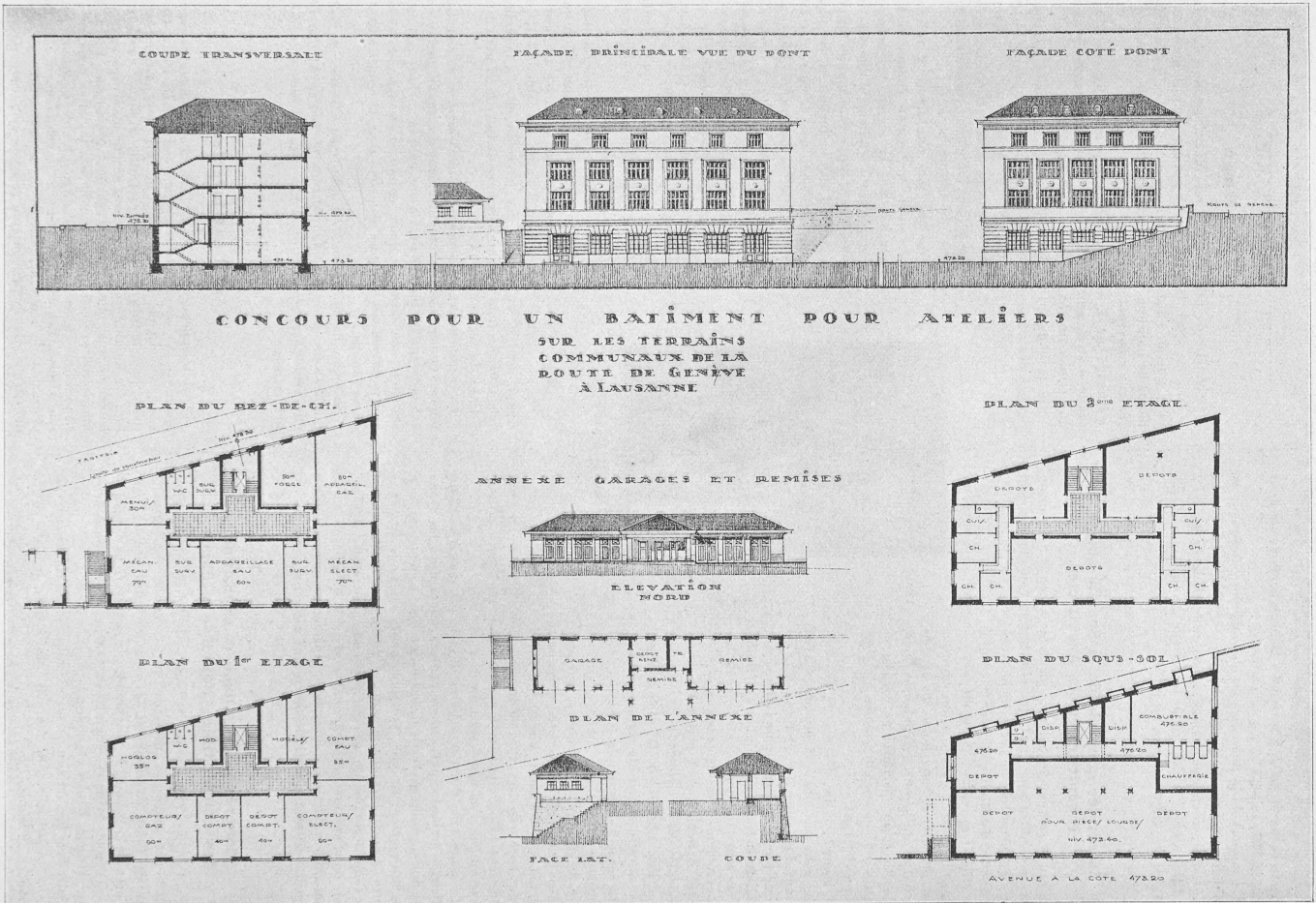
1 er prix : projet « 11 avril », de MM. R. Longchamp & Steiger, architectes, à Lausanne. — Echelle 1 : 600.
