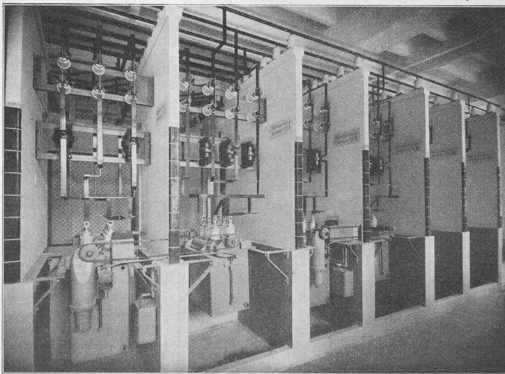
Fig. 39. — Interrupteurs des transformateurs de 800 kVA.
