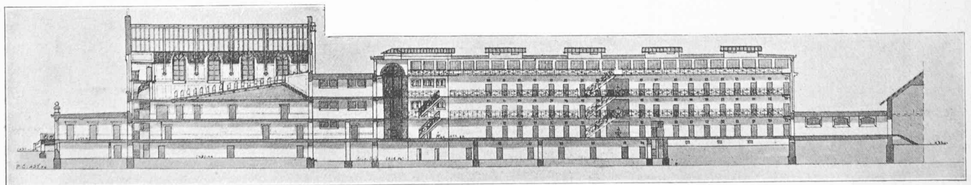
Coupe longitudinale. — 1 : 800.
