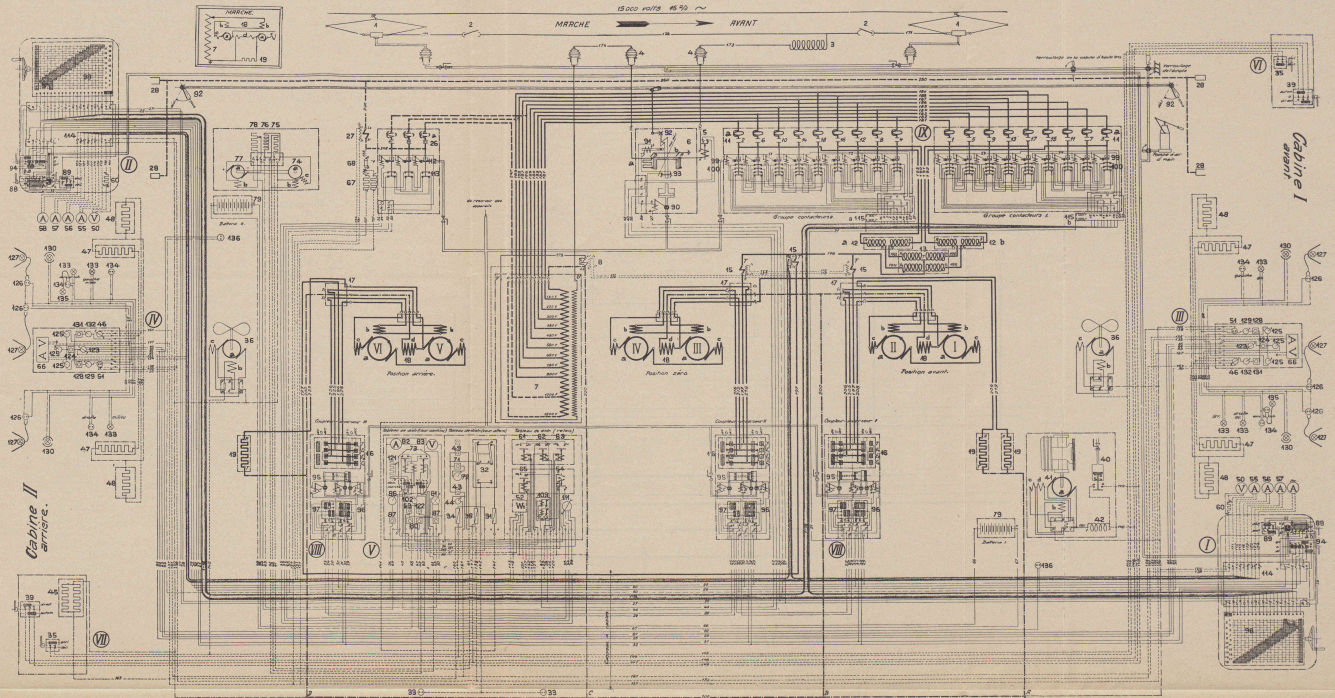
Schéma de la Locomotive électrique type 1C1, Série A* 7/2, des Chemins de fer fédéraux, construite par les Ateliers de Sécheron et la Société suisse pour la construction de locomotives et de machines, à Winterthur.
