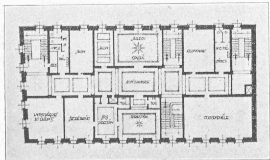
Plan du III e étage. — 1 : 600.
