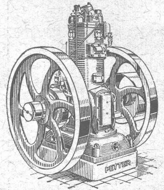
Moteurs Petter à huile lourde.
