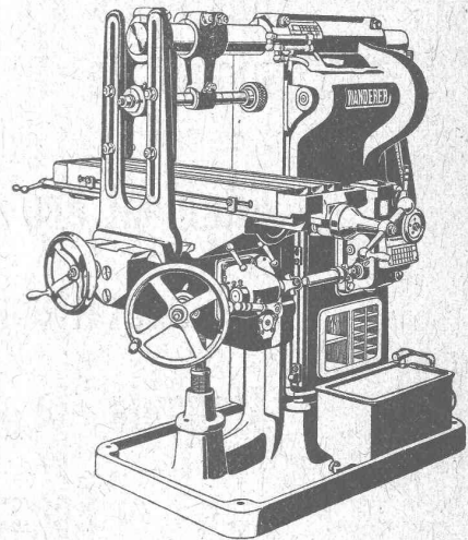
FRAISEUSE - WANDERER
