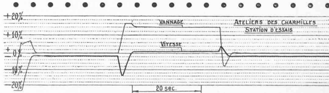
Fig. 12. — Charges et décharges avec statisme négatif.
