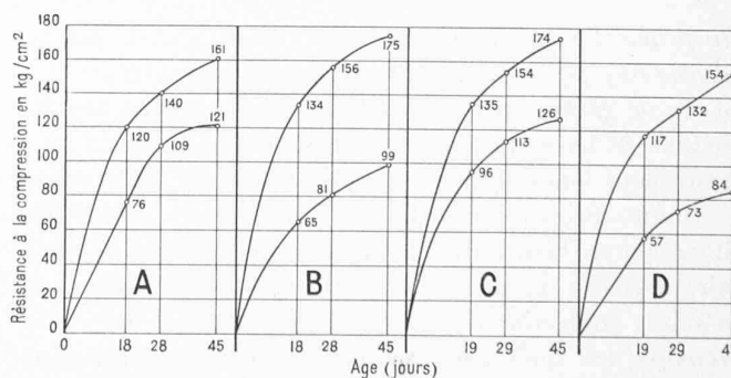
Fig. 2. — Progression du durcissement des bétons obtenus au moyen des matériaux A à D. (Les courbes inférieures correspondent aux bétons des tout-venants, les courbes supérieures au mélange gravier-sable 1 : 2). Dosage : 300 kg. de ciment Portland pour 1200 l. d'un mélange de sable et de gravier. — Résistance propre du ciment I = 408 kg./cm 2 .
