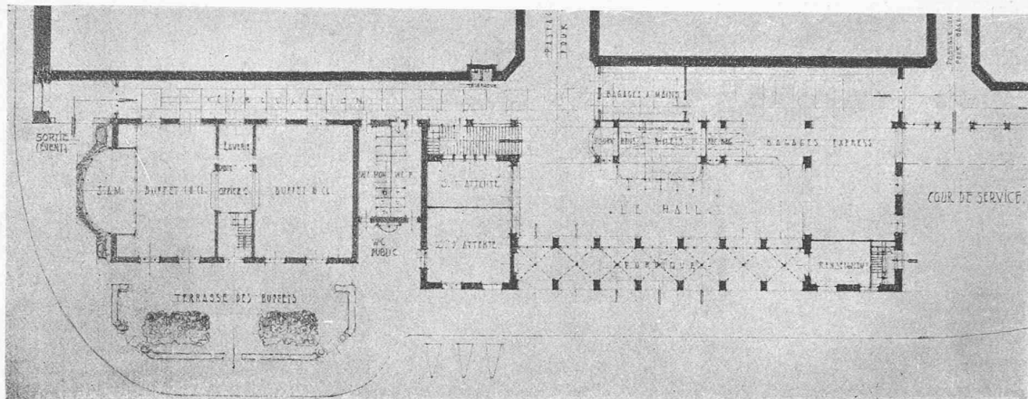
Plan du rez-de-chaussée. — 1 : 600.
