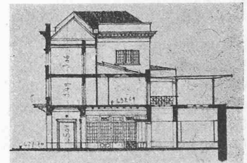
Coupe transversale. — 1 : 600.
