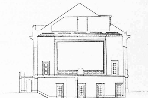
Coupe transversale. — 1 : 400.
