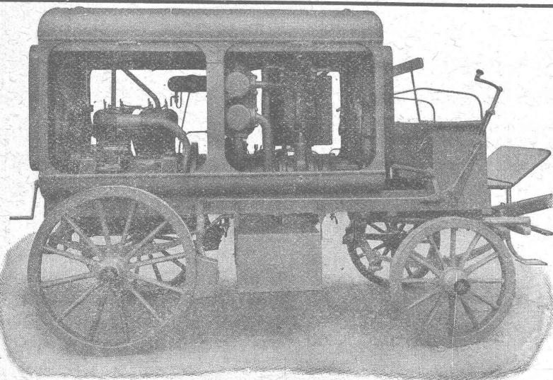
Moto-Compresseur sur char.
