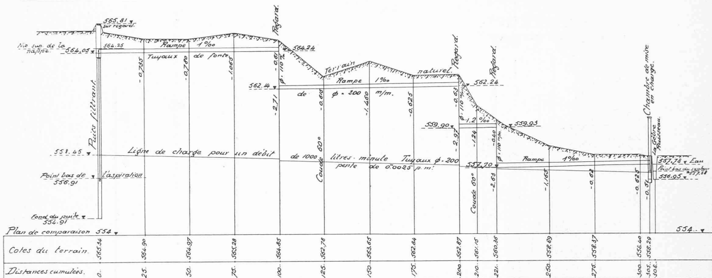
Fig. 3. — Profil en long du syphon.
