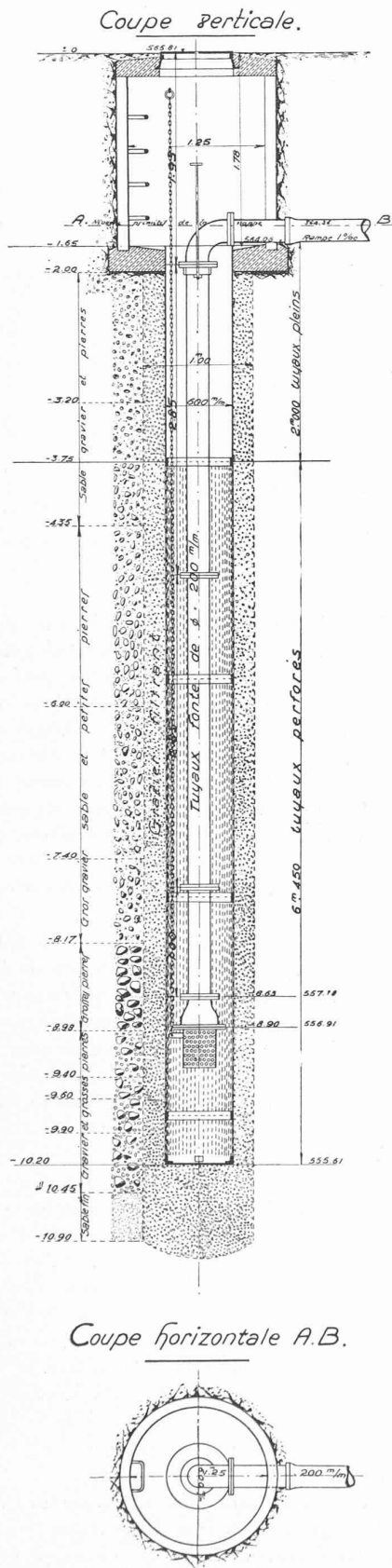
Fig. 1. — Puits filtrant.
