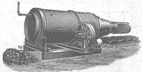
Laveuse-trieuse pour sable.
