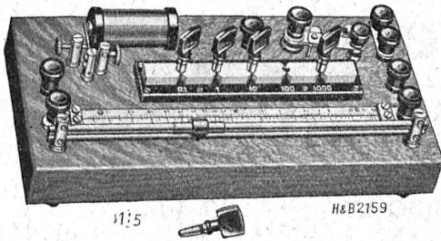
Ponts de résistance à fil et contact curseur de Kohlrusch.
