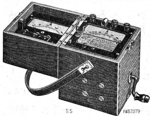
1:5 H&B2079 Mesureur d'isolement avec voltmètre.
