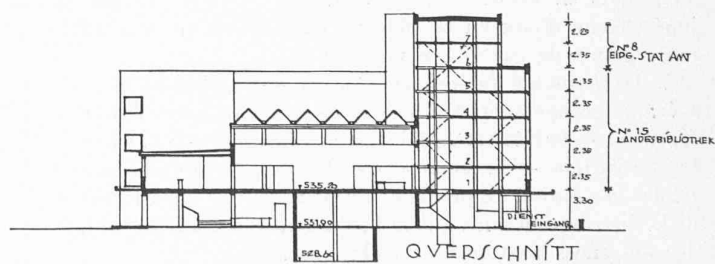
Coupe. — 1 : 660.
