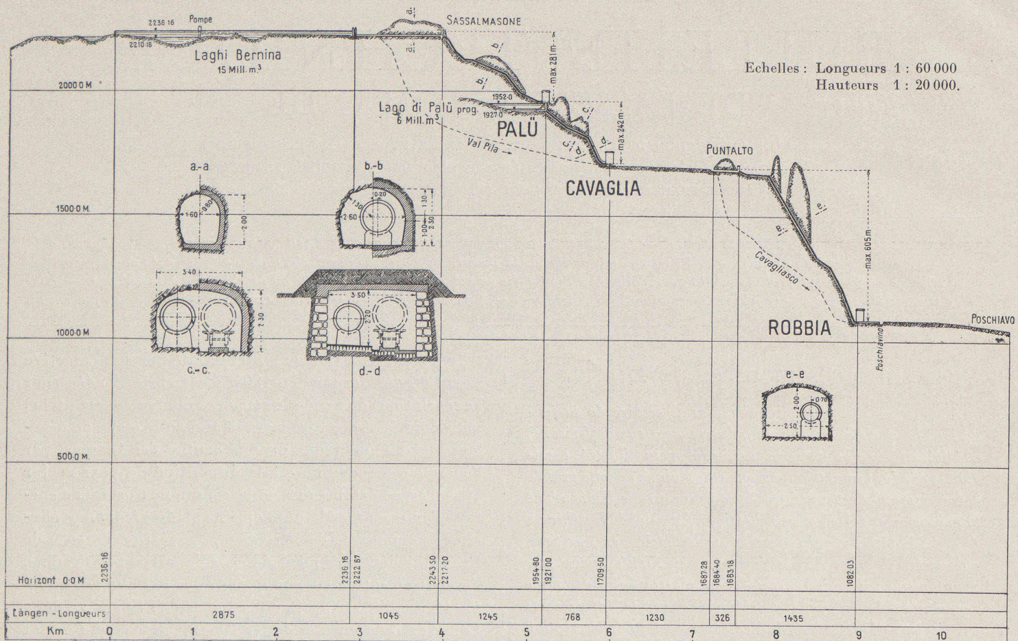
Fig. 1. — Profil en long général de l'aménagement des
