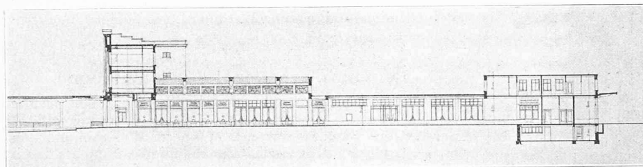
Coupe longitudinale. — 1 : 800.
