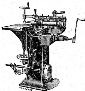
Mortaiseuse.
